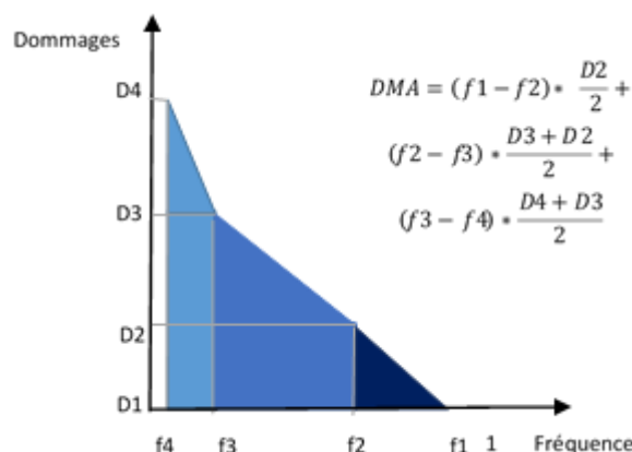
Figure 9 – Représentation et calcul du dommage moyen annuel
