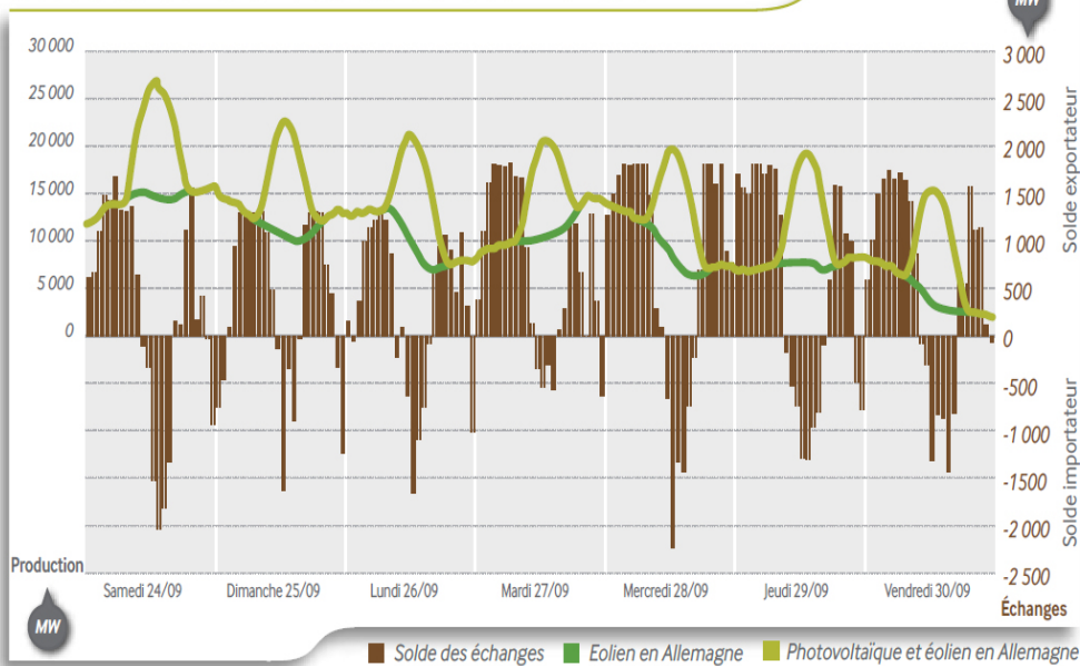
Évolution comparée du solde des échanges sur la frontière franco-allemande et de la production éolienne et photovoltaïque en Allemagne
